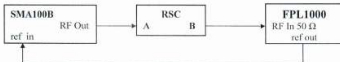
Рисунок 5 – Структурная схема соединения СИ для определения абсолютной погрешности измерений уровня мощности входного сигнала из-за переключения ослабления аттенуатора СВЧ
