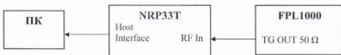
Рисунок 12 – Структурная схема соединения СИ для определения абсолютной погрешности установки уровня выходного синусоидального сигнала минус 10 дБ (1 мВт)
