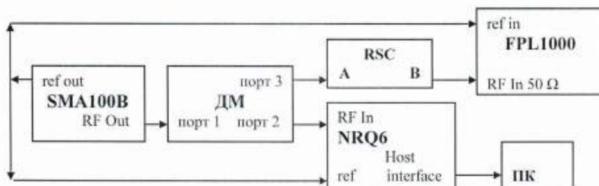
Рисунок 6 – Структурная схема соединения СИ для определения абсолютной погрешности измерений отношения мощностей в диапазоне измерений уровней мощности
