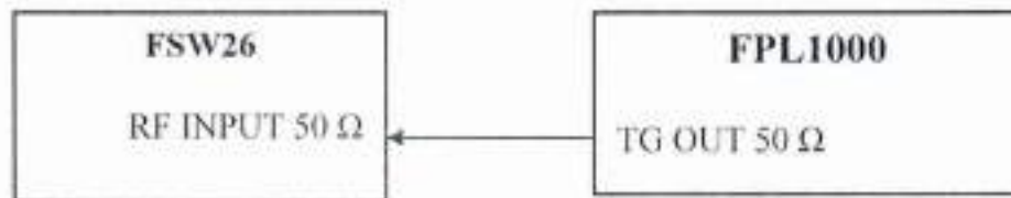
Рисунок 11 – Структурная схема соединения СИ для определения уровня фазовых шумов на частоте 1 ГГц
